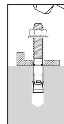
Ankerbout inslaan
