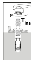
Aandraaimoment toepassen
